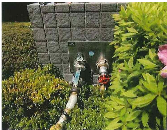
送水口
